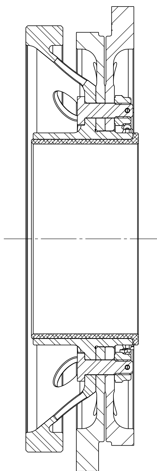
SECTION A-A
