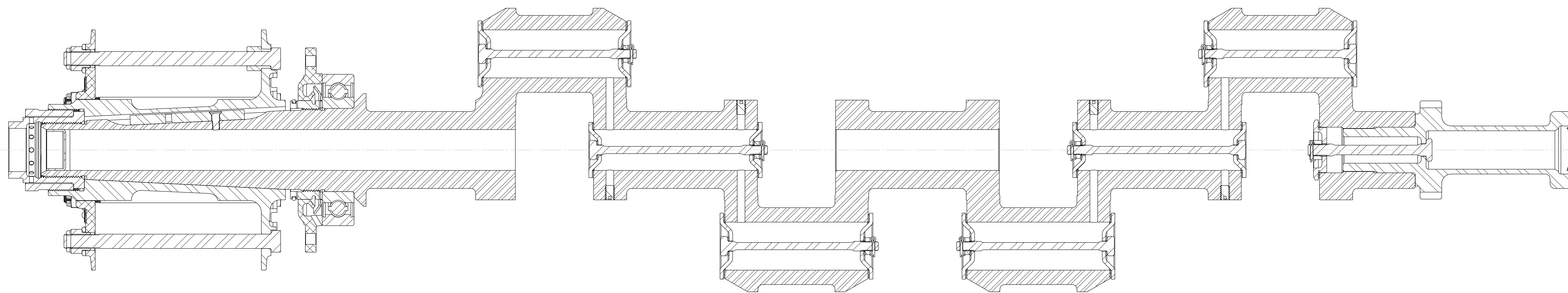
SECTION A-A
